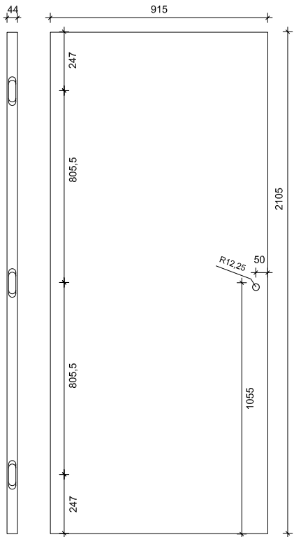
Porte cieche battenti ferramentate
