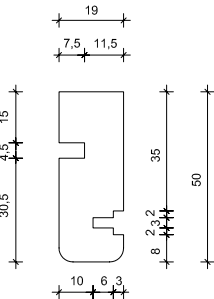
Profilo architrave - Bino’s 100
