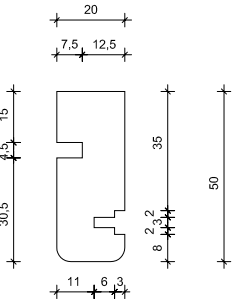
Profilo architrave - Bino’s 108
