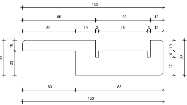
PORTASPAZZOLINO PER SCORREVOLE ESTERNO
