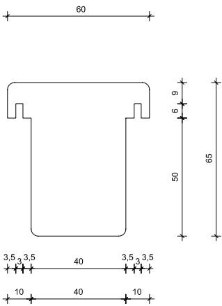
Separatore sopraluce
