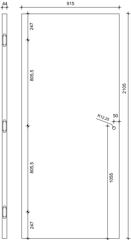
Porte cieche battenti ferramentate
