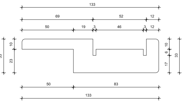
PORTASPAZZOLINO PER SCORREVOLE ESTERNO
