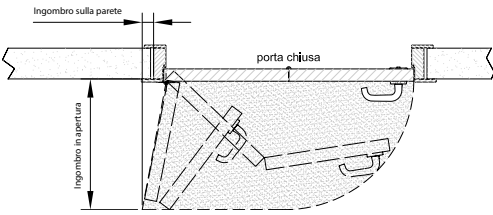
Schema porta Compack 90° - esempio di porta SX
