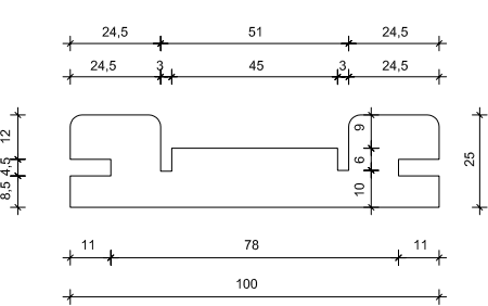
Montante telaio - Bino’s 100
