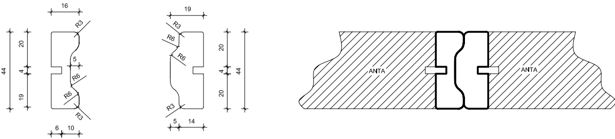
SCAMBIO BATTUTA PER ANTA DOPPIA BATTENTE
