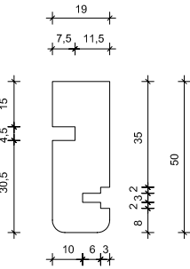
Profilo architrave - Bino’s 100
