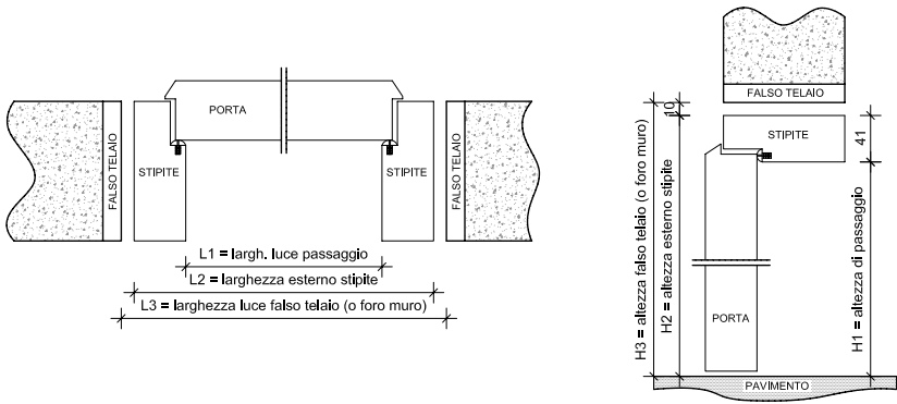
PORTA BATTENTE MONTATA SU PARETE IN MURATURA sezione verticale e orizzontale
