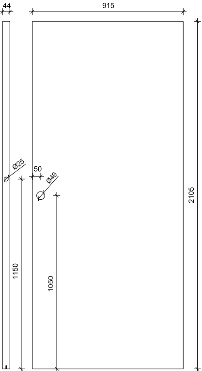
Porte cieche scorrevoli ferramentate
