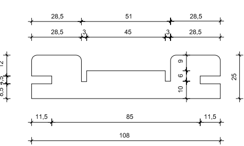
Montante telaio - Bino’s 108
