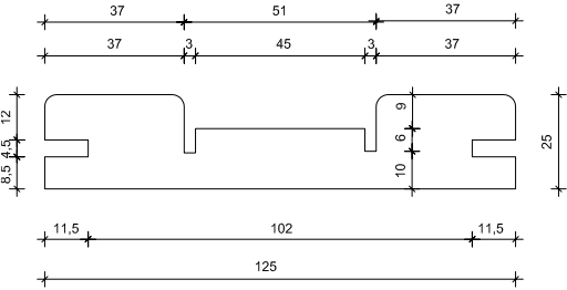
Montante telaio - Bino’s 125
