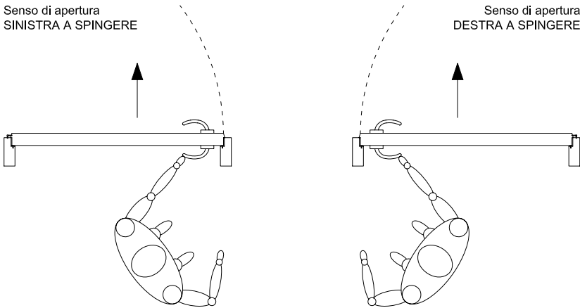
SENSO DI APERTURA PORTE sezione verticale e orizzontale
