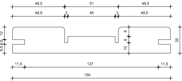
Montante telaio - Bino’s 150
