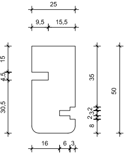
Profilo architrave - Bino’s 125
