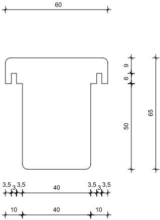
Separatore sopraluce
