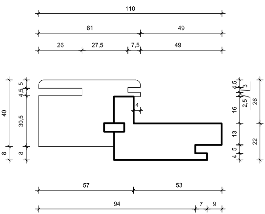
Stipite per traverso di porta pieghevole compact
