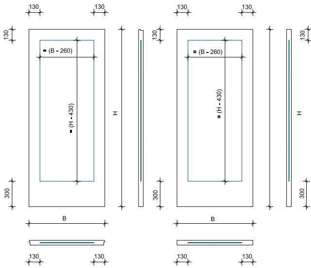
Dimensioni foro vetro porta standard
