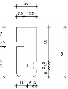
Profilo architrave - Bino’s 108
