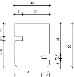
Profilo architrave - Bino’s 150
