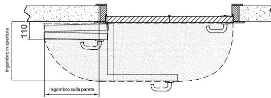
Schema porta Compack 180° - esempio di porta SX
