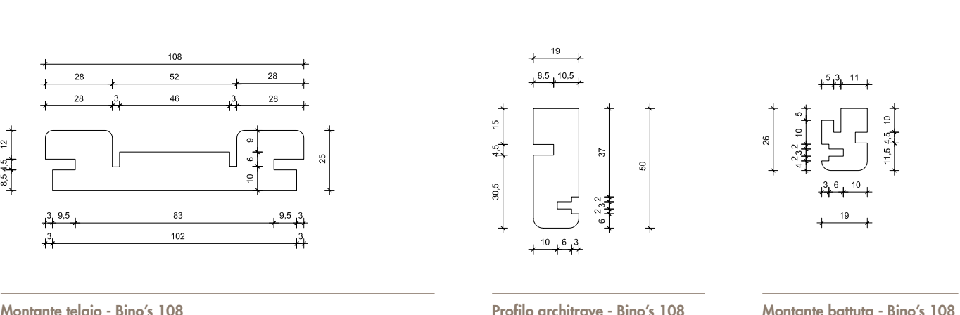
Montante telaio - Bino's 108
