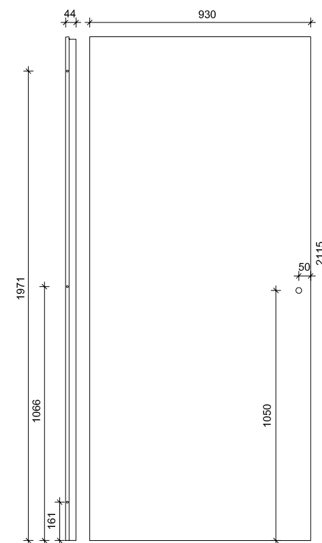
Porte cieche battenti ferramentate
