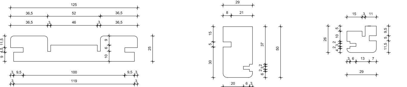
Montante telaio - Bino's 125
