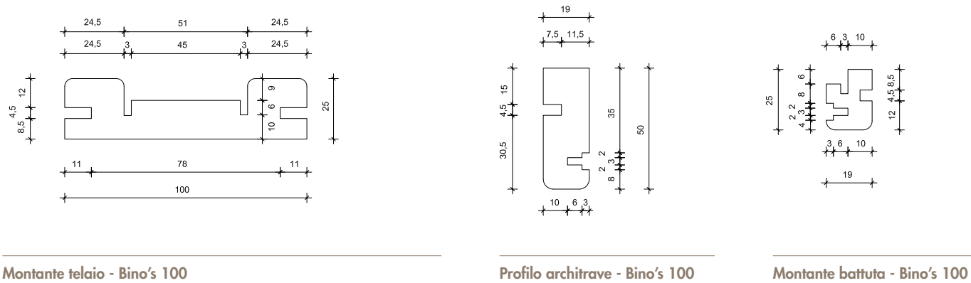
Montante telaio - Bino's 100
