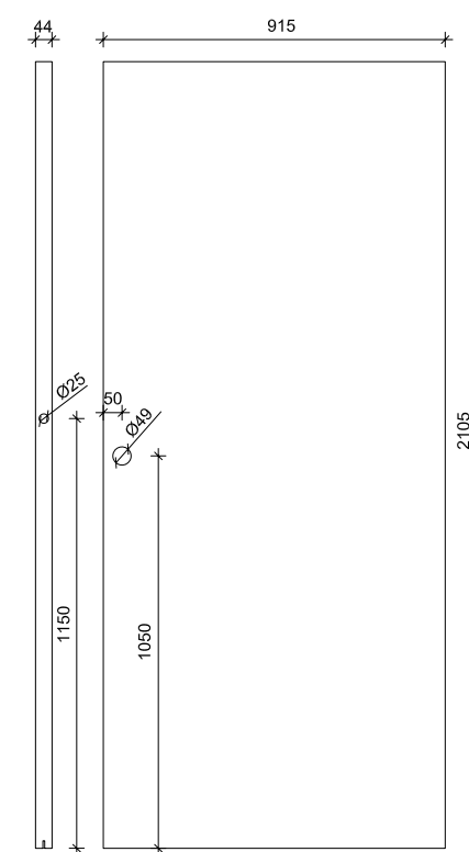
Porte cieche scorrevoli ferramentate
