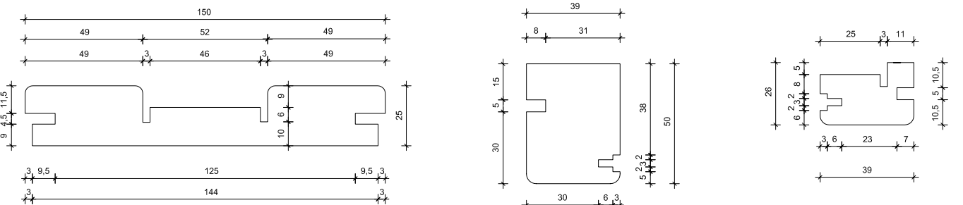
Montante telaio - Bino's 150
