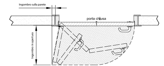
Schema porta Compack 90° - esempio di porta SX
