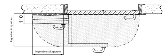
Schema porta Compack 180° - esempio di porta SX
