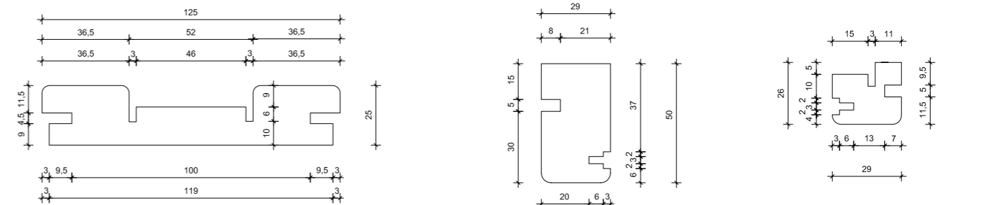
Montante telaio - Bino's 125
