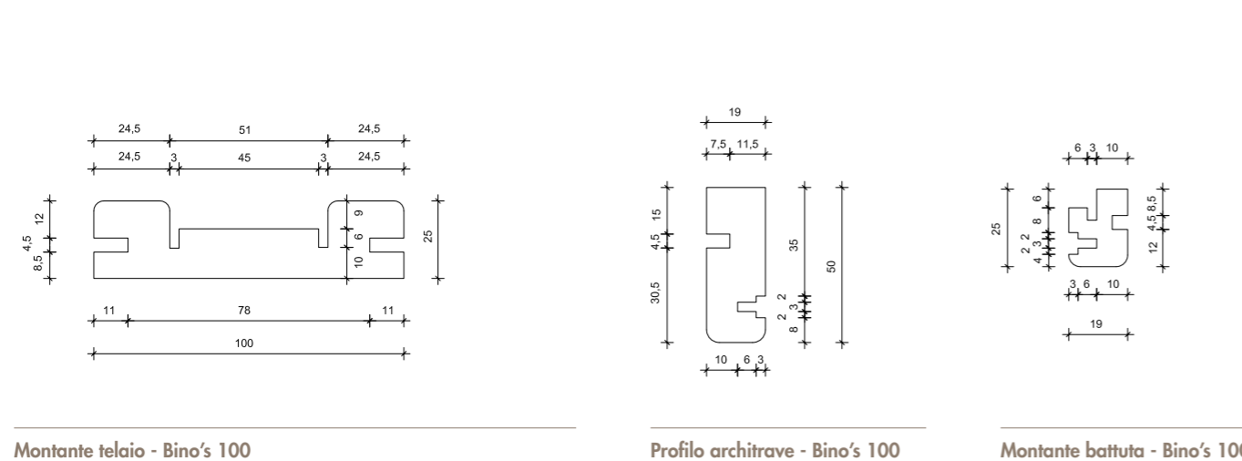
Montante telaio - Bino's 100
